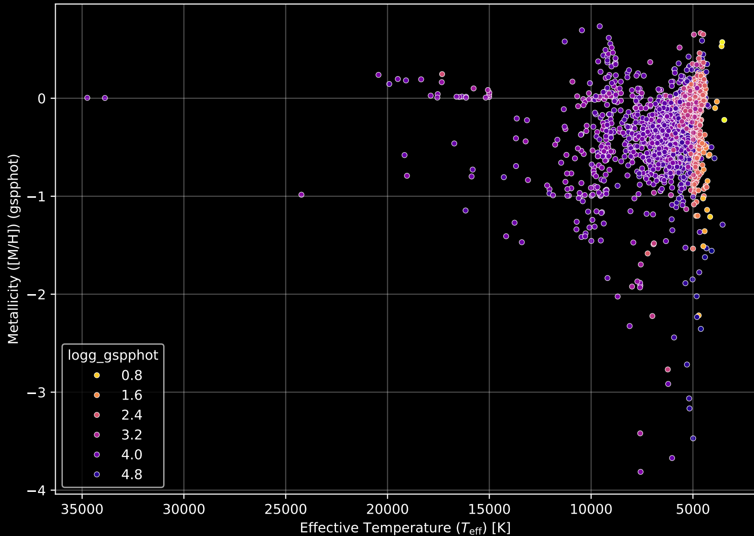
GALAH DR4 Field: [-3] Stellar Population Parameters (n= 1982)
