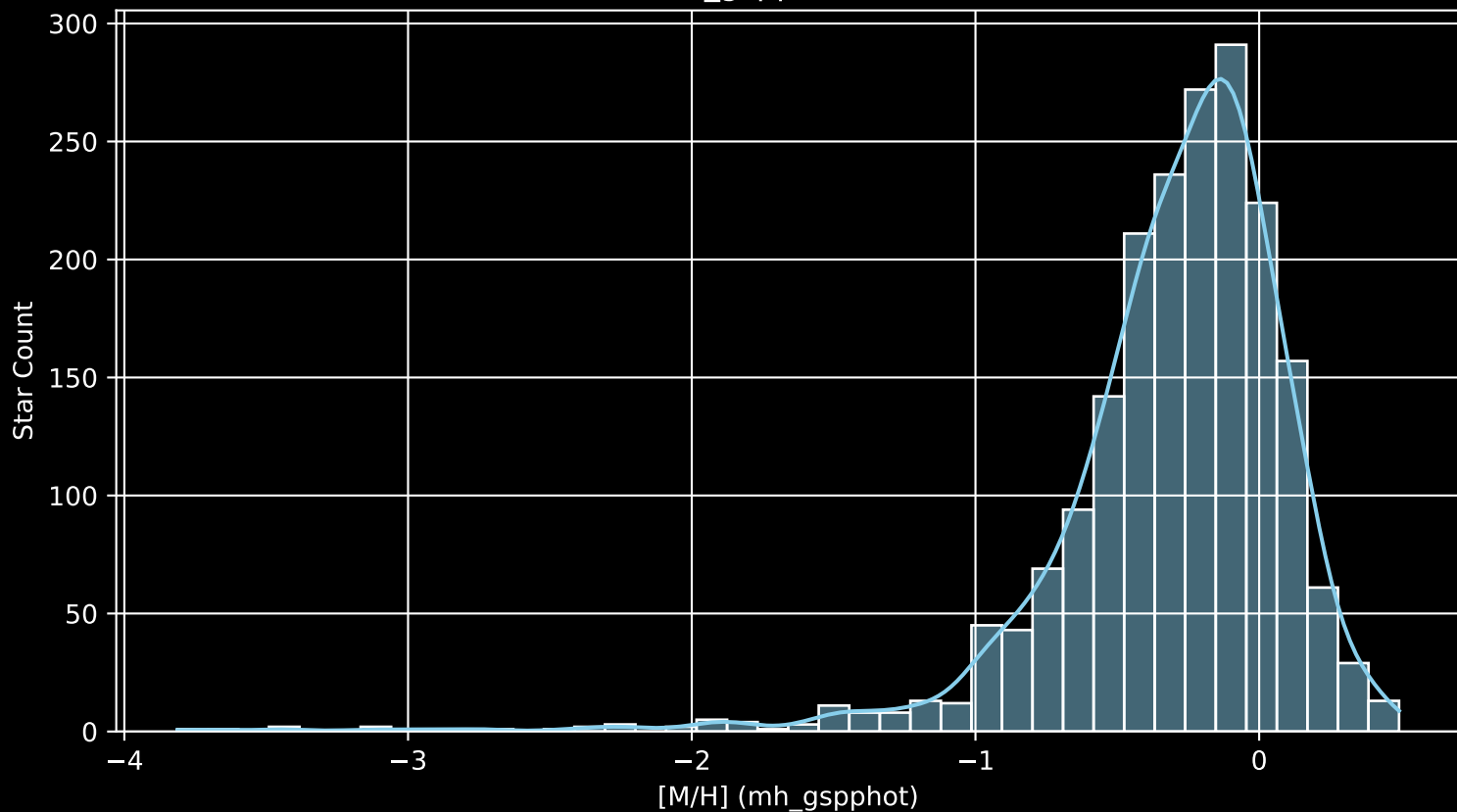
GALAH DR4 Field: [-3] [M/H] (mh_gspphot) (n= 1969)
